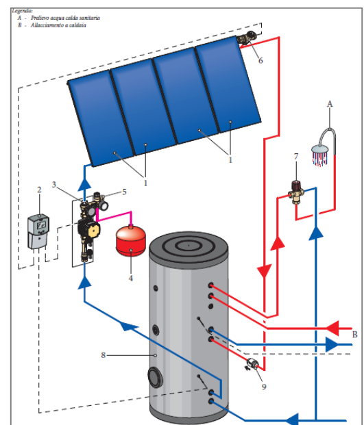
Skeme installimi i nje Kit INOX SOL 500 ErP
